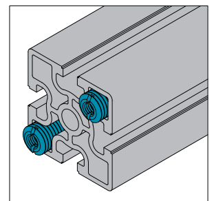
变径螺栓M16/M8 用于60系列型材四角孔-14x14(M16)
