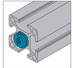
变径螺栓M12/M6 用于30系列型材中心孔-Φ10(M12)
