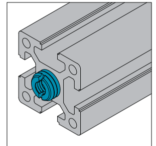
变径螺栓M14/M8 用于40系列/45系列/50系列/60系列型材中心孔-Φ12(M14)
