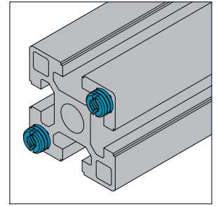
变径螺栓M10/M6 用于45系列型材四角孔-8x8(M10)
