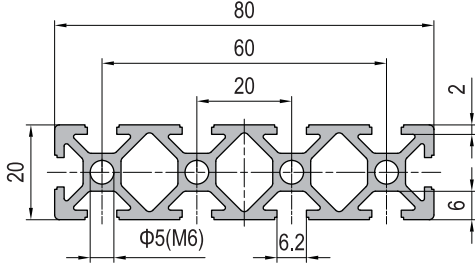
PG20 20x80 10 slots
