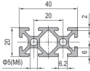
PG20 20x40 6 slots
